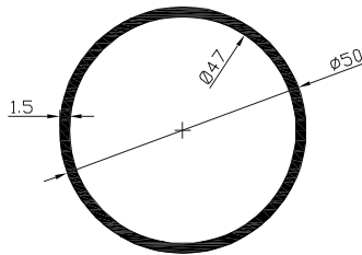
Kod-Code VM405 Profil-Profil 50 Boru Profil-Ø50 Pipe Profile Ağırlık-Weight 0.616kg/m
