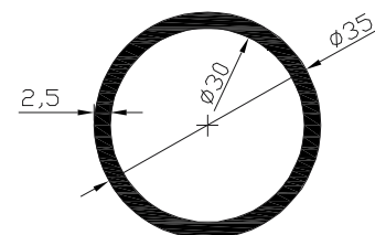
Kod-Code VM418 Profil-Profil 35 Boru Profil-Ø35 Pipe Profile Ağırlık-Weight 0.689kg/m
