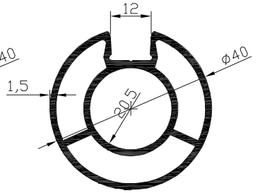
Kod-Code VM412 Profil-Profil 40 Dikme -Ø40 Poppet Ağırlık-Weight 0.872kg/m
