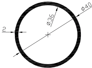
Kod-Code VM406 Profil-Profil 40 Boru Profil-Ø40 Pipe Profile Ağırlık-Weight 0.644kg/m
