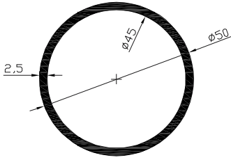
Kod-Code VM401 Profil-Profil 50 Boru Profil-Ø50 Pipe Profile Ağırlık-Weight 1.01kg/m
