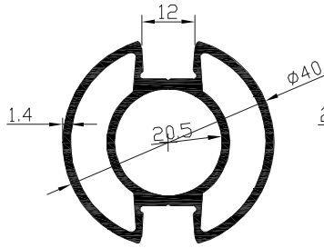
Kod-Code VM409 Profil-Profil 40 Dikme -Ø40 Poppet Ağırlık-Weight 0.802kg/m
