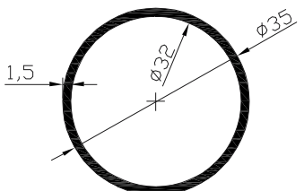
Kod-Code VM420 Profil-Profil 35 Boru Profil-Ø35 Pipe Profile Ağırlık-Weight 0.426kg/m
