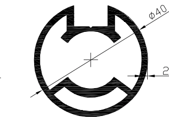
Kod-Code VM414 Profil-Profil 40 Dikme -Ø40 Poppet Ağırlık-Weight 0.99kg/m
