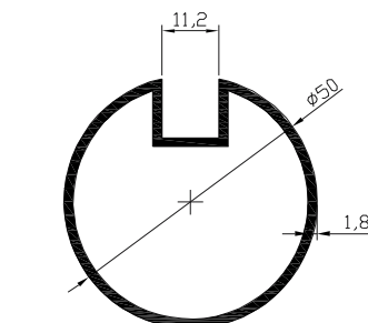
Kod-Code VM417 Profil-Profil 50 Boru Profil-Ø50 Pipe Profile Ağırlık-Weight 0.857kg/m
