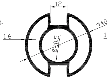
Kod-Code VM411 Profil-Profil 40 Dikme -Ø40 Poppet Ağırlık-Weight 0.948kg/m
