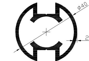
Kod-Code VM413 Profil-Profil 40 Dikme -Ø40 Poppet Ağırlık-Weight 0.942kg/m
