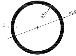
Kod-Code VM403 Profil-Profil 50 Boru Profil-Ø50 Pipe Profile Ağırlık-Weight 1.196kg/m
