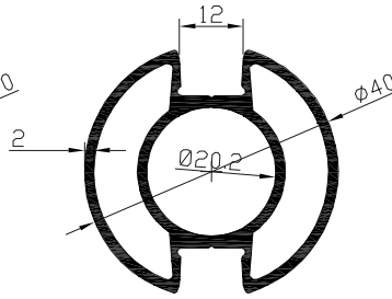
Kod-Code VM410 Profil-Profil 40 Dikme -Ø40 Poppet Ağırlık-Weight 1.24kg/m
