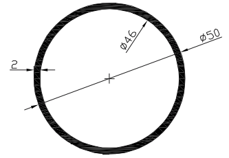
Kod-Code VM404 Profil-Profil 50 Boru Profil-Ø50 Pipe Profile Ağırlık-Weight 0.815kg/m
