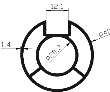
Kod-Code VM415 Profil-Profil 40 Dikme -Ø40 Pipe Profile Ağırlık-Weight 0.830kg/m
