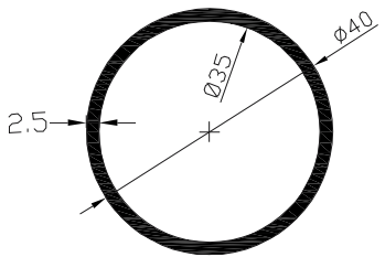
Kod-Code VM408 Profil-Profil 40 Boru Profil-Ø40 Pipe Profile Ağırlık-Weight 0.797kg/m
