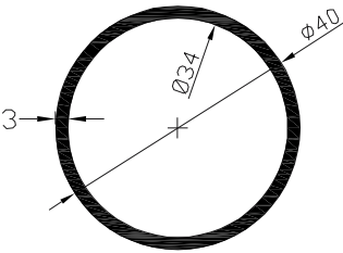
Kod-Code VM407 Profil-Profil 40 Boru Profil-Ø40 Pipe Profile Ağırlık-Weight 0.942kg/m
