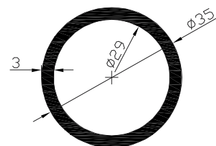
Kod-Code VM419 Profil-Profil 35 Boru Profil-Ø35 Pipe Profile Ağırlık-Weight 0.813kg/m
