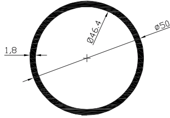
Kod-Code VM402 Profil-Profil 50 Boru Profil-Ø50 Pipe Profile Ağırlık-Weight 0.734kg/m
