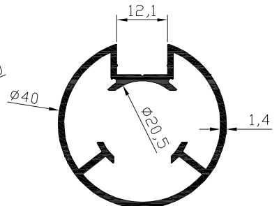
Kod-Code VM416 Profil-Profil 40 Boru Profil-Ø40 Pipe Profile Ağırlık-Weight 0.670kg/m
